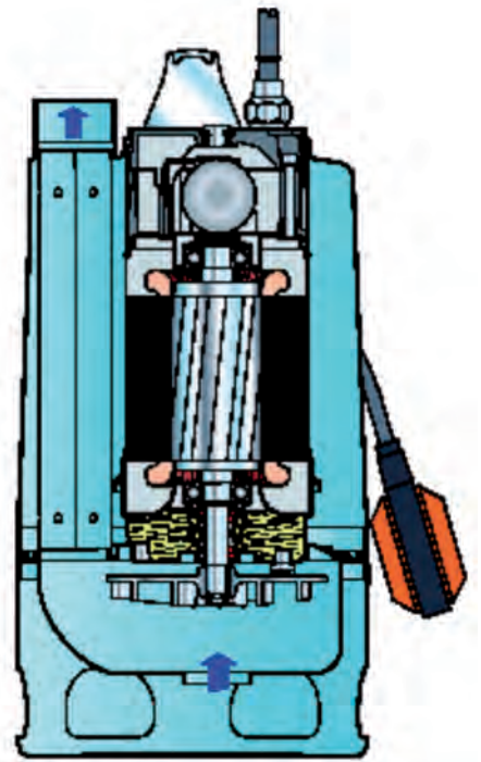
Pompa DOMO RX® in sezione.
